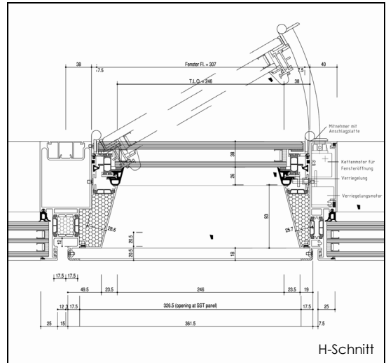
Elektromotorischer Lüftungsflügel der Bürofassade
